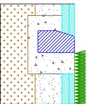
SECCION - DETALLE DE COLOCACION DE BORDILLOS
