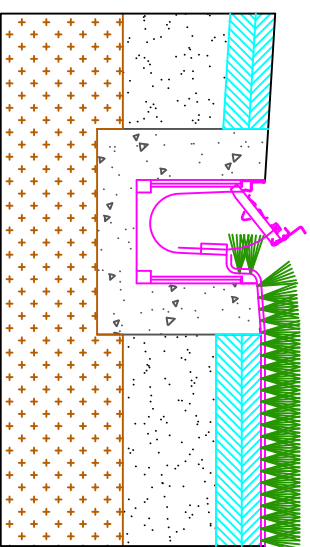
SECCION - DETALLE DE COLOCACION DE CANALETA EN LATERALES DEL TERRENO DE JUEGO
